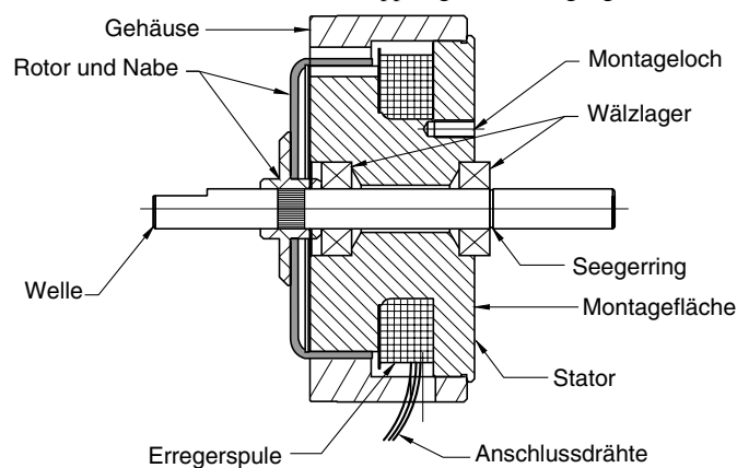
Bild 1. Hysteresebremse
